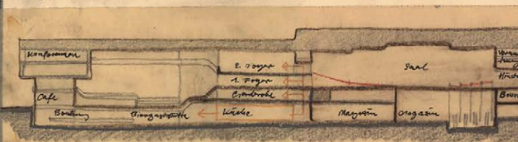
Längsschnitt 1:500
